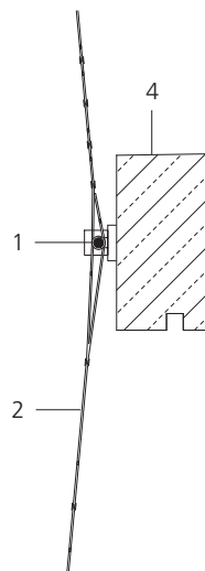
Détail. Vue de face. Echelle 1:10 1 Ralingue Ø 12 mm, inox EN 1.4401 2 Filet fils Ø 3 mm, inox EN 1.4401 3 Plot de guidage cylindrique, inox EN 1.4404 4 Dalle de la coursière, béton préfabriqué
