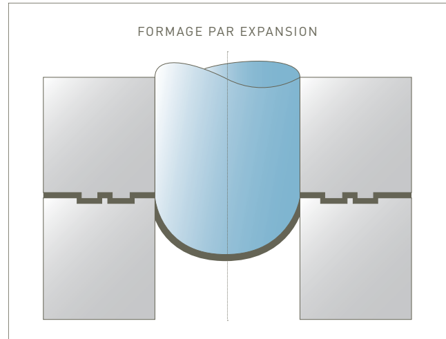
En formage par expansion, la partie emboutie devient plus mince.
