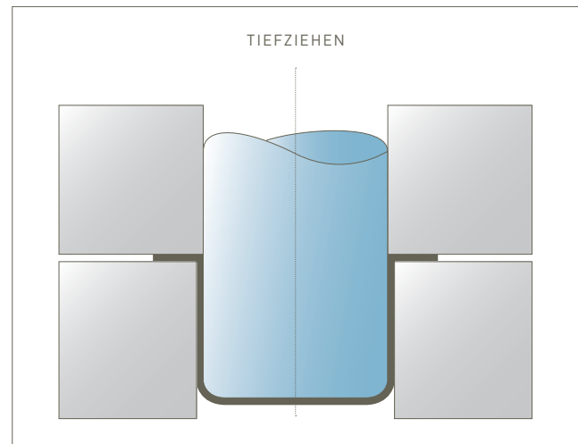
Beim Umformen unterscheidet man „Tiefziehen“ und „Streckziehen“, bei letzterem wird die Platine vom Niederhalter festgehalten.
