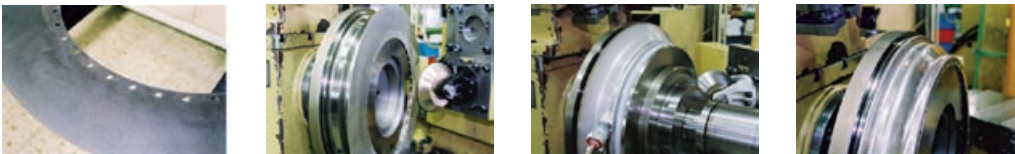
Drücken des Außenrings. Während des Umformprozesses erhöht sich die Festigkeit des nichtrostenden Stahls. Hierdurch wird die Felge robuster gegenüber Stößen.
